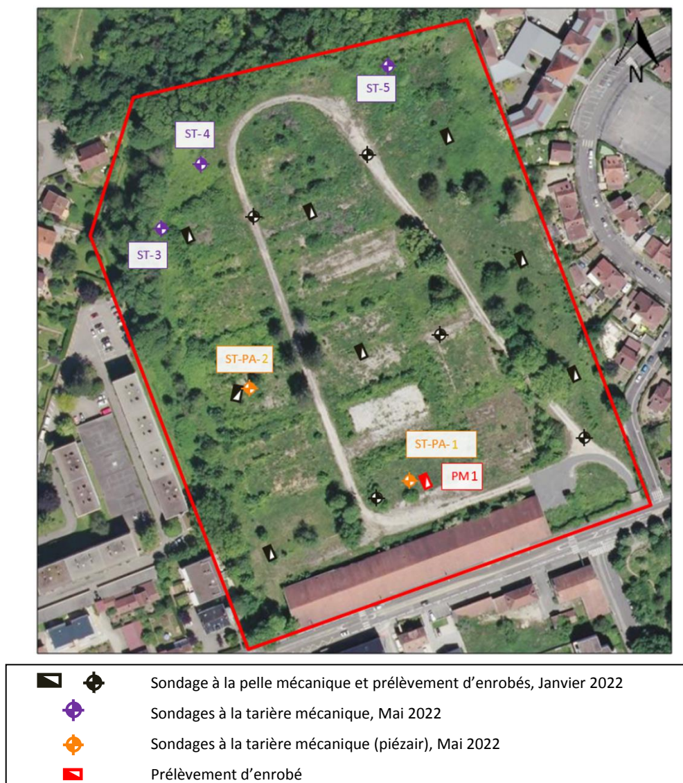
Figure 13 : Plan du point de prélèvement d'enrobé
